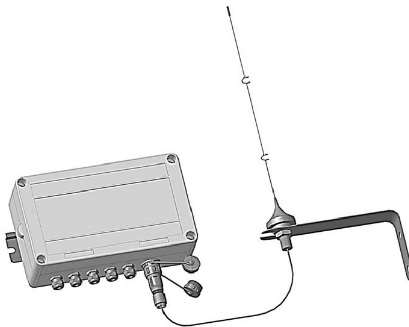
Рис.1. Внешний вид преобразователя измерительного «ВЗЛЕТ АС» исполнения АСДТ.
